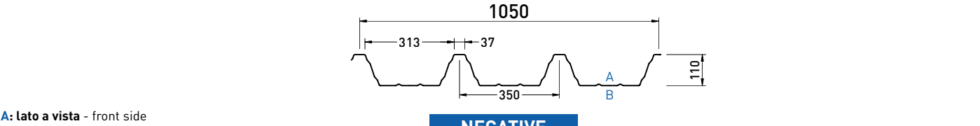
A: lato a vista - front side B: lato non a vista - back side
